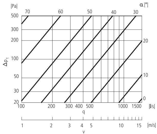
Ø400
