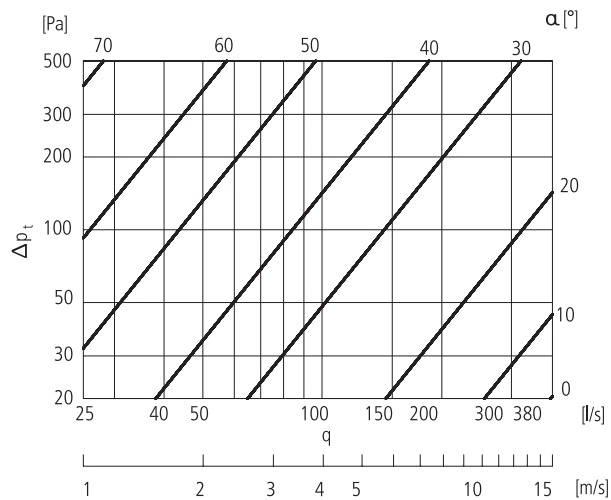
Ø180
