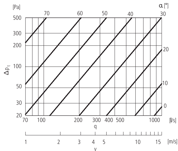
Ø300
