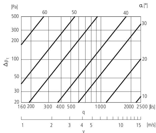
Ø500
