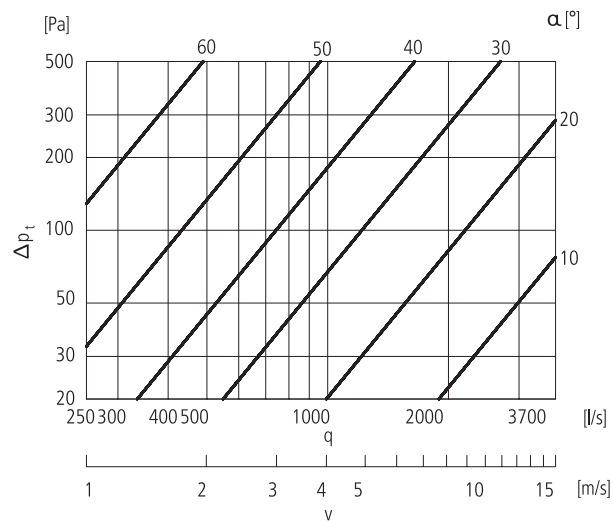
Ø560
